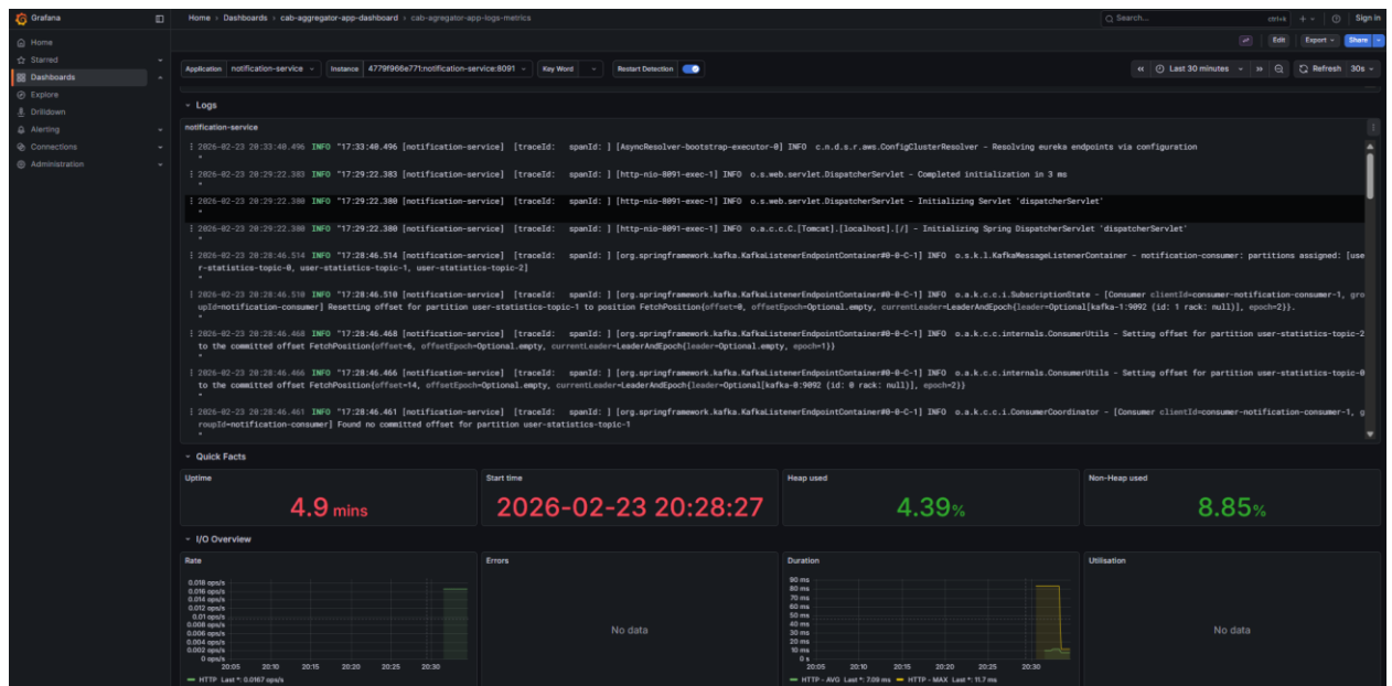
Рисунок 1.7 – Веб-интерфейс Grafana
