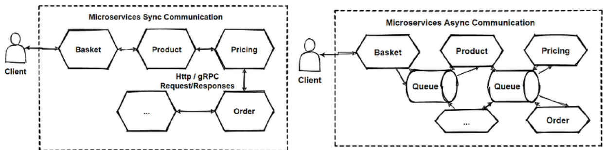
Рисунок 1.5 – Сравнение синхронного и асинхронного способа взаимодействия в микросервисной архитектуре [6]
